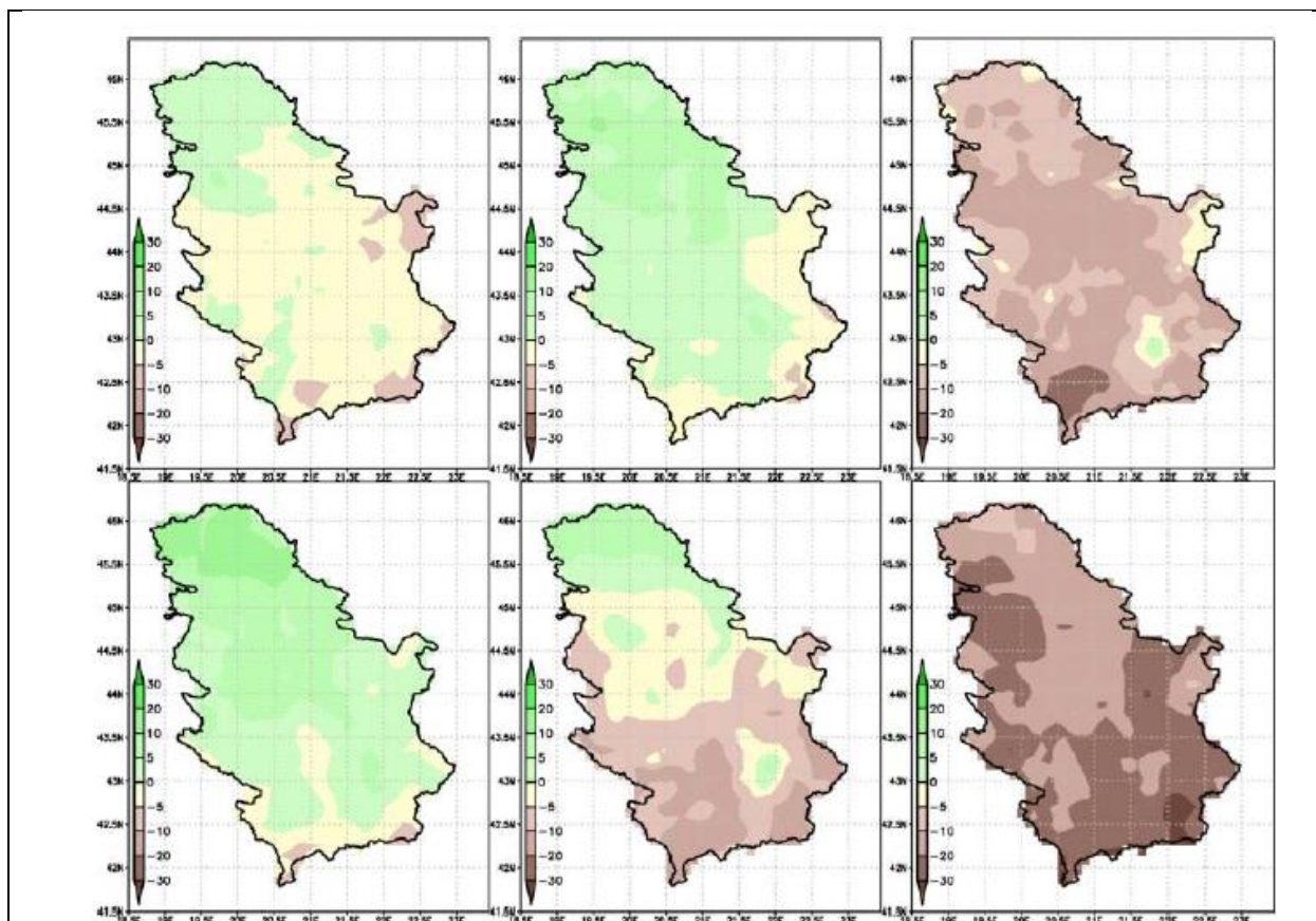
Слика III.27: Одступање средње суме падавина (%) (Извор: Осмотрене промене климе у Србији и пројекције будуће климе на основу различитих сценарија будућих емисија70)
